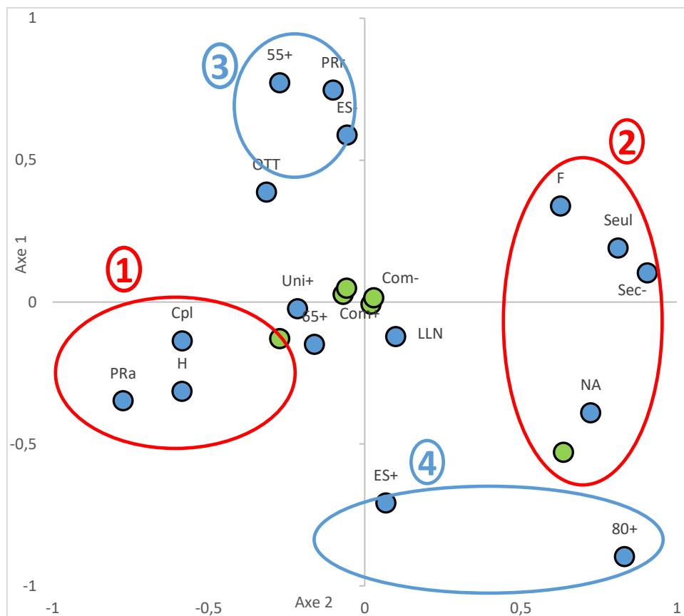
Figure 18. Projection des variables sur le premier plan orthogonal de l'analyse en composante multiple.
